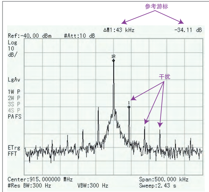
图4. 在打开荧光灯的环境中对915MHz射频信号进行空中测量。所示为43KHz(电子照明镇流器的工作频率)的调制边带
