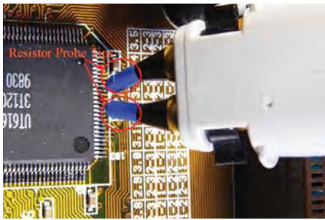
Figura 8-4. Todas as pontas de prova da série N2750A da InfiniiMode, da série 1156A-58A e da série InfiniiMax usam essa tecnologia de acessórios com amortecimento para oferecer uma performance ótima, porém flexível.
