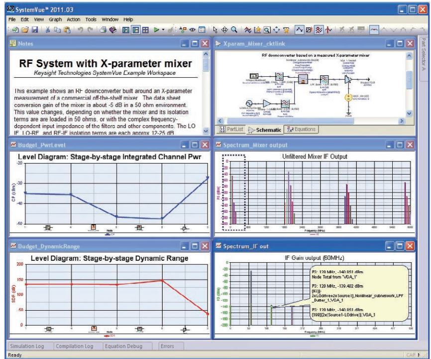
図3. Spectrasysは、I/Q不整合、双方向伝搬、非線形性、周波数応答、リーケージ成分、DCからミリ波までのスペクトラム全体を考慮して、個々の信号や雑音要因をトラッキングします。これらを、グラフから直接対話形式で数秒で調べることができます。
