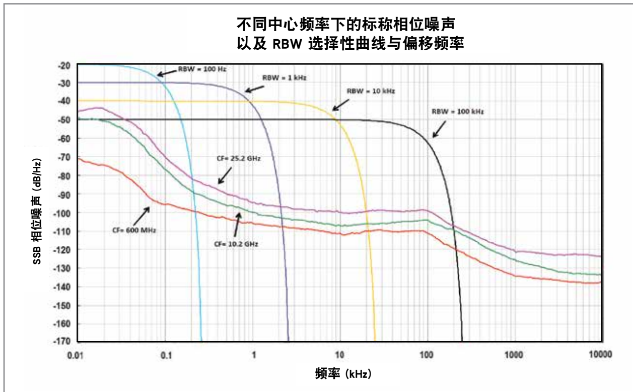
图 1. CXA 不同中心频率上的标称相位噪声
